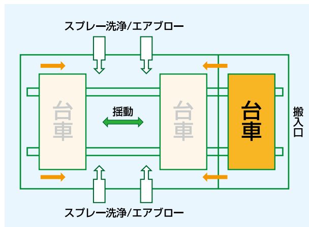
洗浄機を上から見たイメージ図
