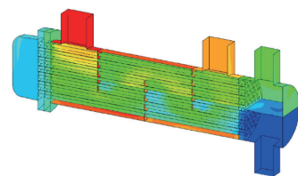
熱交換器の流体解析・熱応力解析
